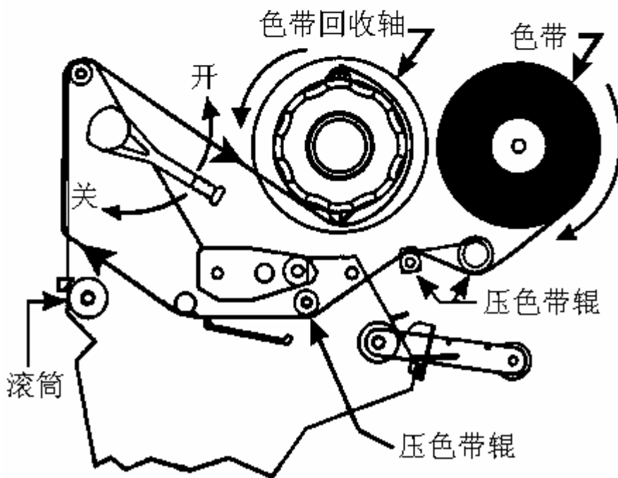
Z170XII 和 Z220XIII 色带安装图
