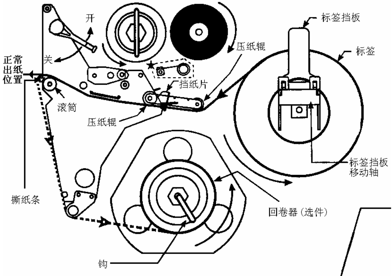
图 5 标签安装图
